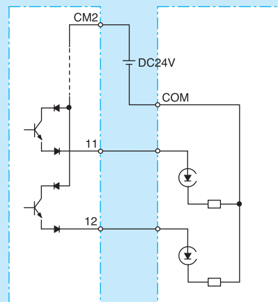
SJ700 Hitachi EH-150 series PLC Input Module EH-XD16
