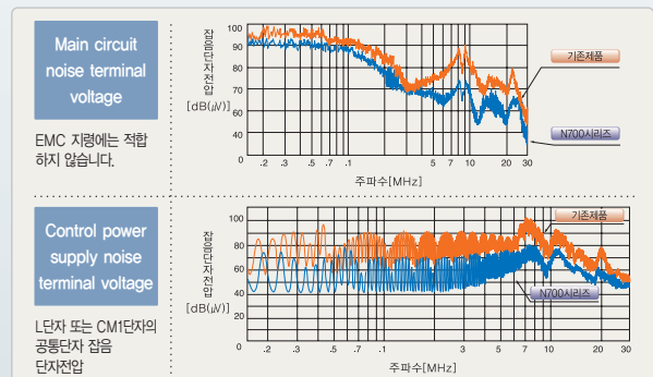
[ 인버터에서 발생하는 노이즈 및 누설전류 감소 효과 ]
